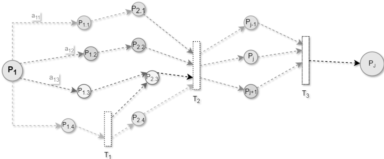
Рис. 1. Схема процесів функціонування кольорової мережі Петрі з умовними позначенням етапів проекту , вузлів переходів та спрямованих дуг між ними
